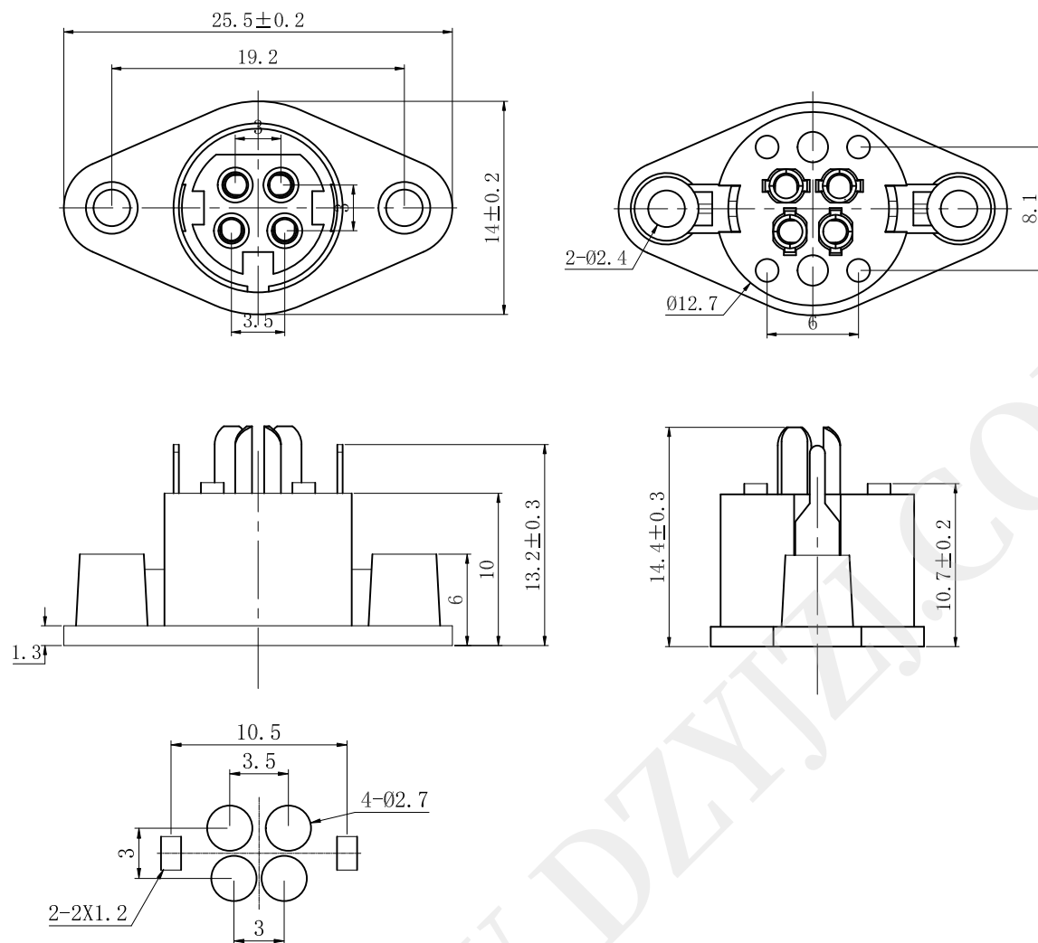
PCB板安装孔图
