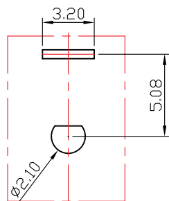
线路板开孔尺寸图
