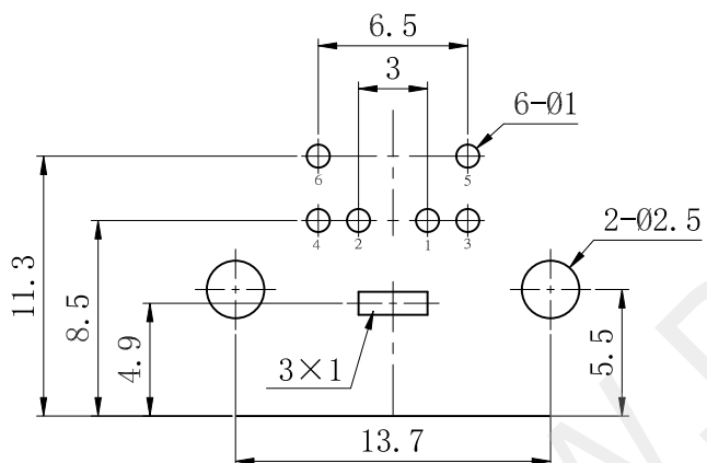
PCB板安装孔图
