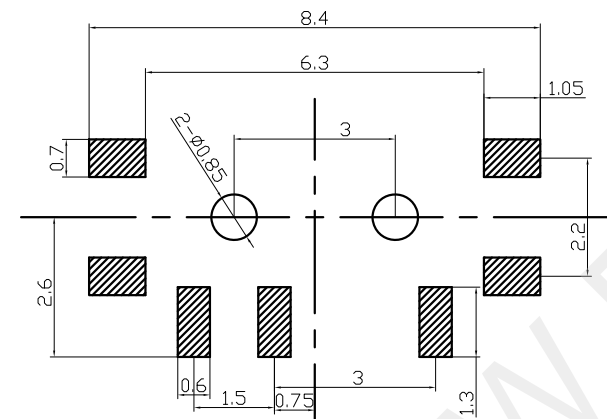
安装参考图
