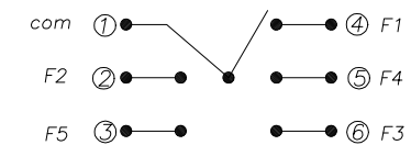
电路图
