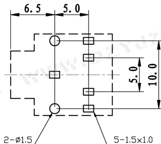
线路板安装尺寸示意图
