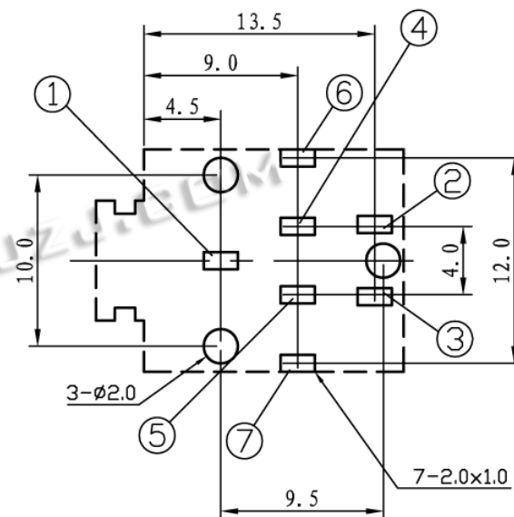
线路板按装尺寸示意图
