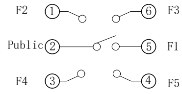
电路图
