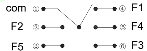
电路图
