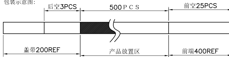
包装示意图:
