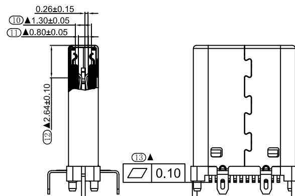
截面 A-A
