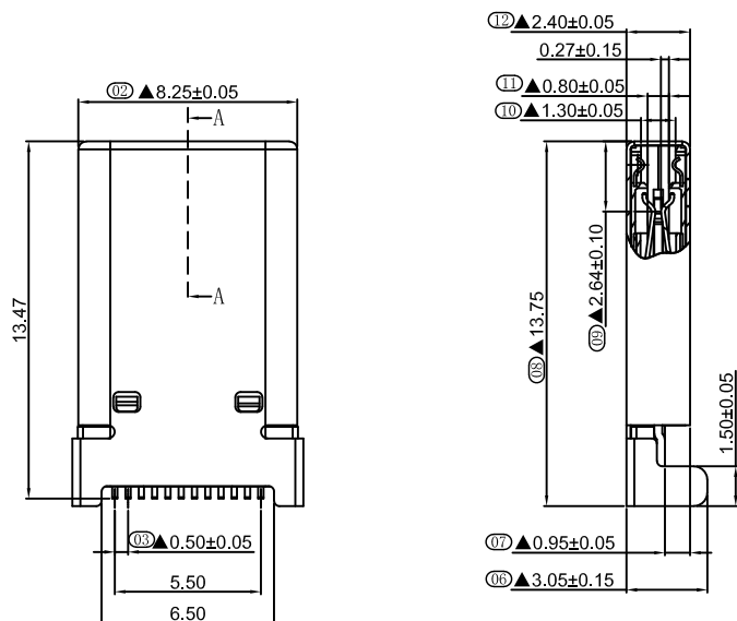
截面 A-A
