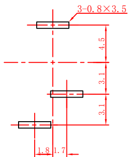
印制电路板开孔尺寸
