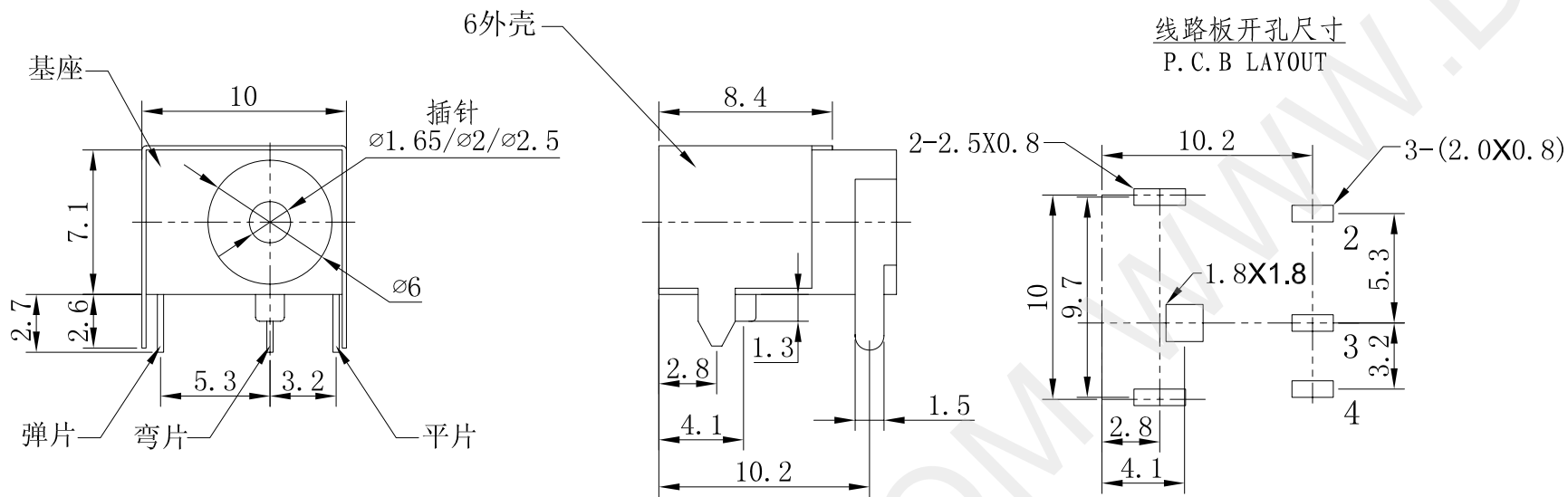
按点示意图 SCHEMATIC
