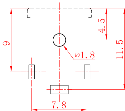
电路板开孔尺寸
