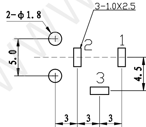
线路板安装示意图
