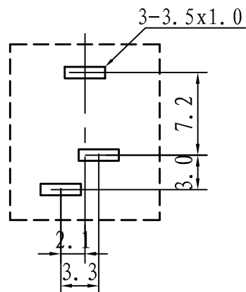
线路板安装尺寸示意图
