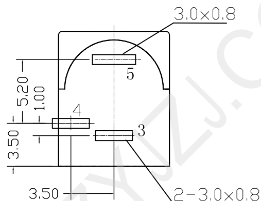
电路板开孔尺寸 TOP VIEW
