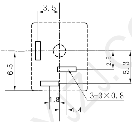
线路板开孔尺寸
