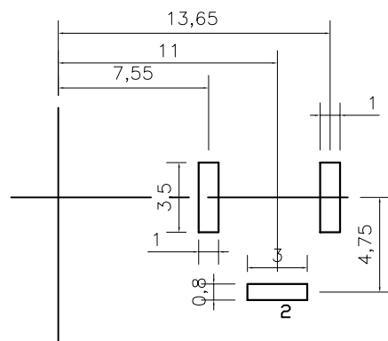
推荐PCB板开孔尺寸
