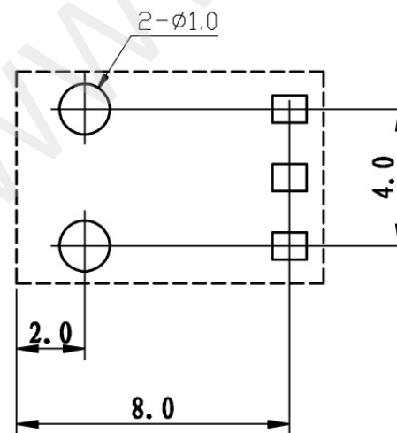
线路板安装尺寸示意图
